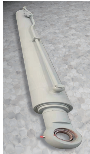
抛落迦油缸
